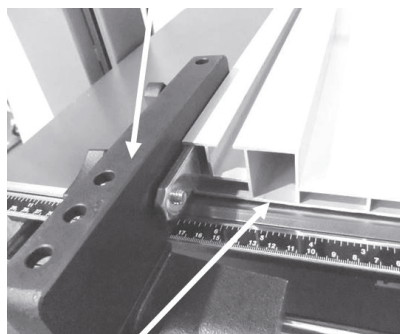
Pravítko v horizontální pozici
